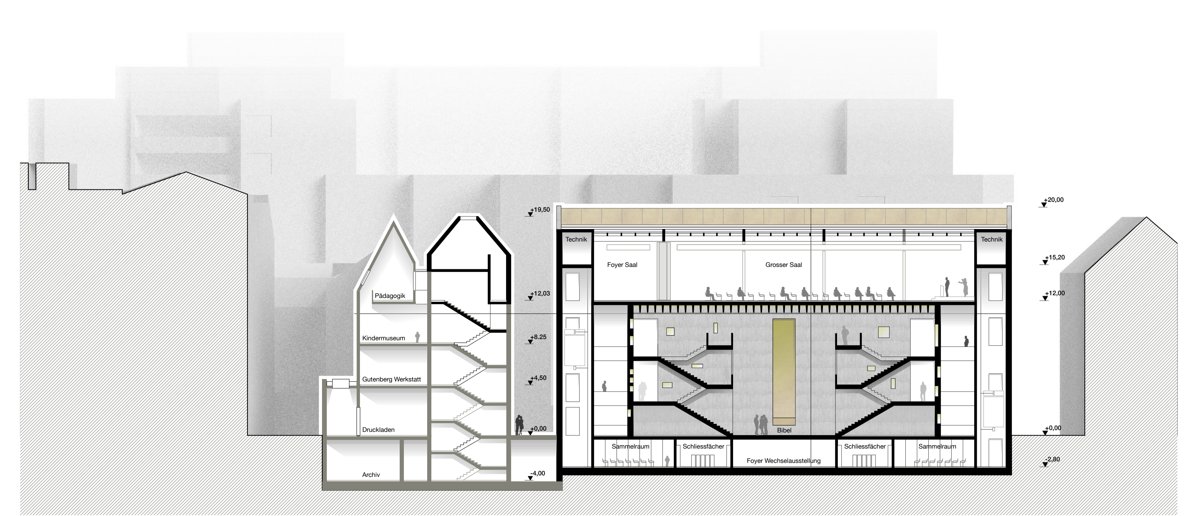
SCHNITT B-B 1:200
