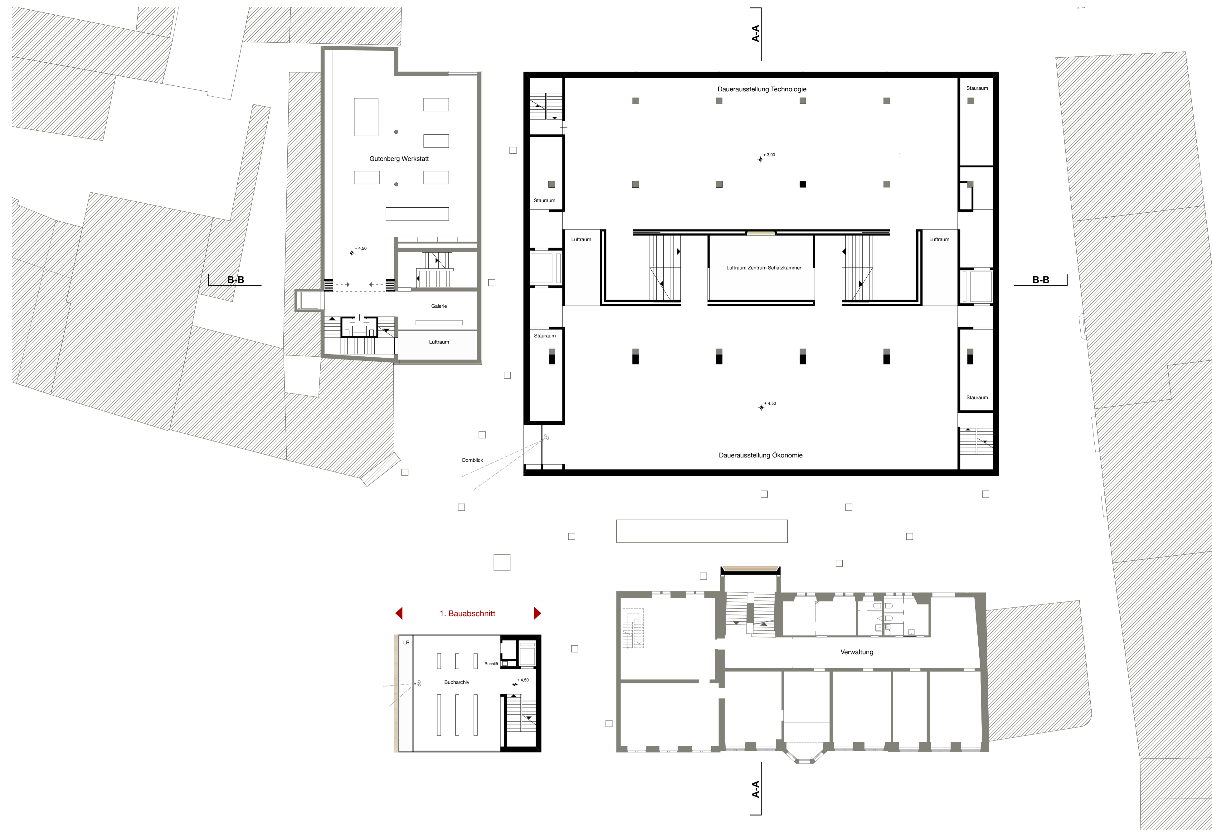
1. OBERGESCHOSS 1:200
