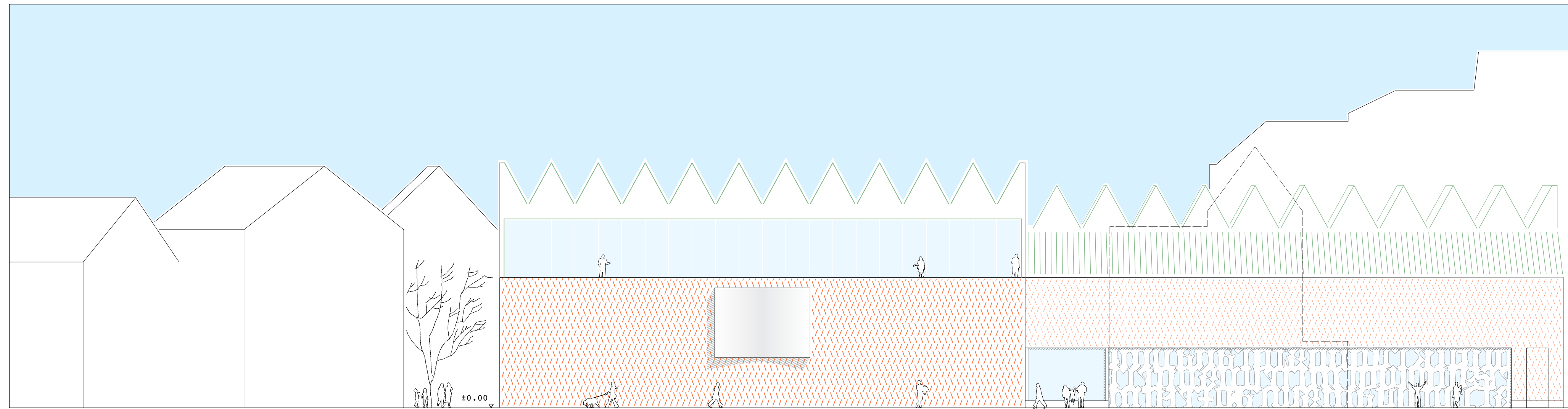
ansicht nord 1:200
