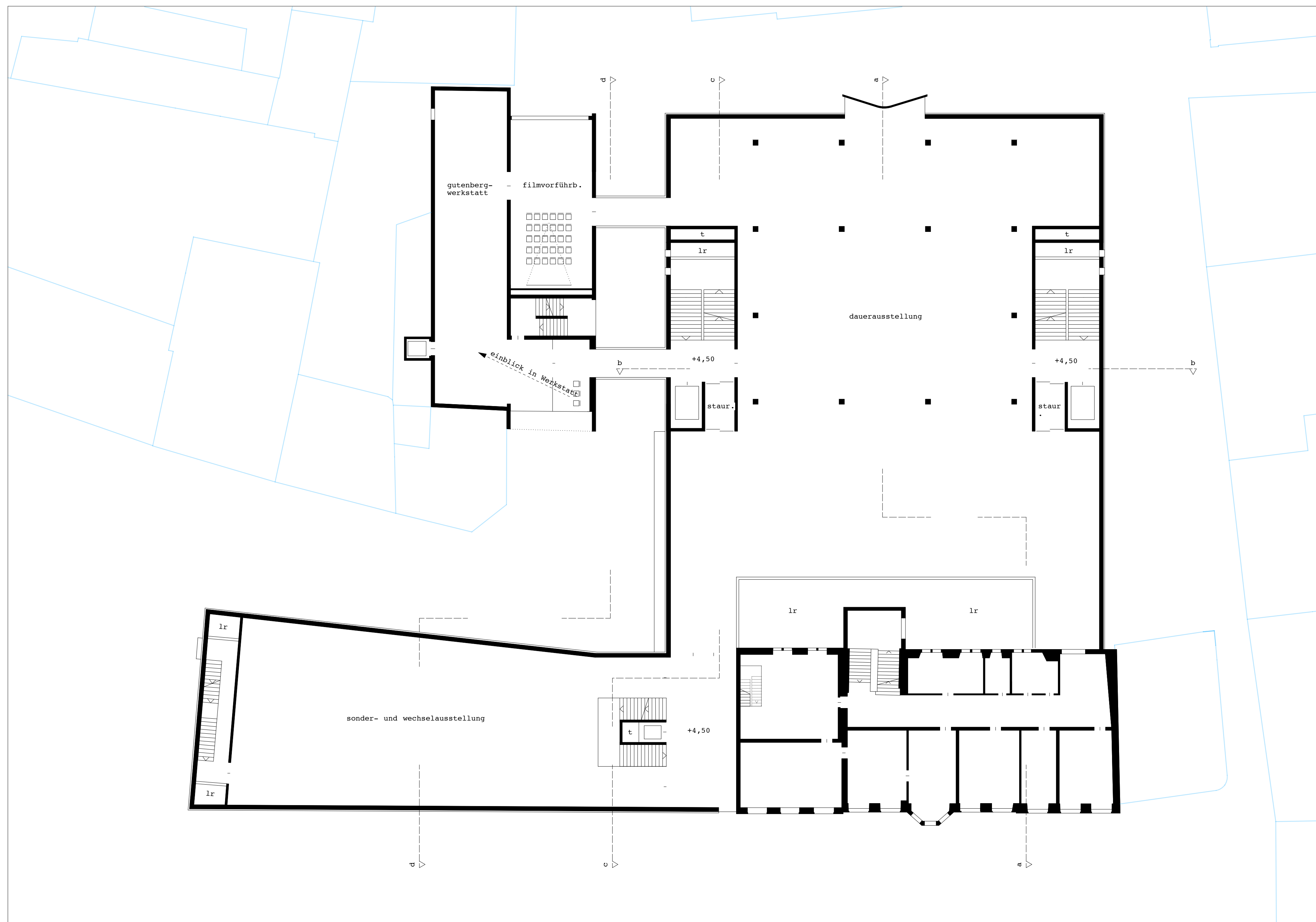
1.obergeschoss 1:200
